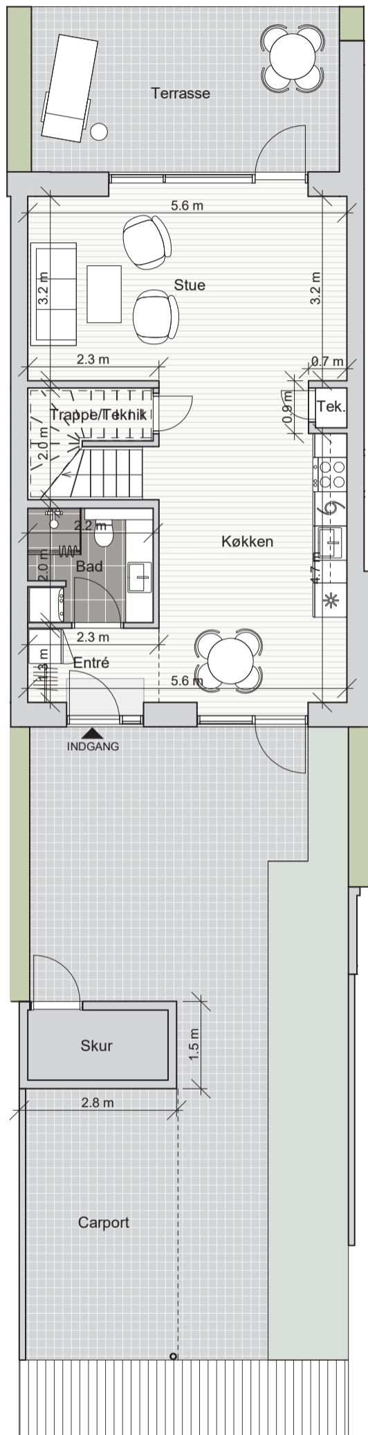
Stueplan
